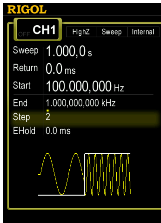
Bild 6-3 Sprung Wobbelsignal
