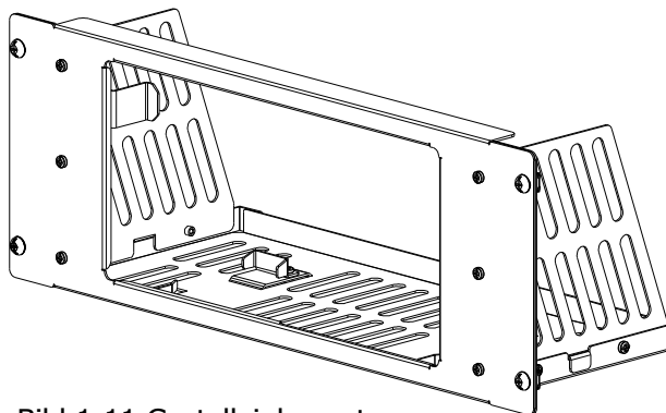
Bild 1-11 Gestelleinbausatz
