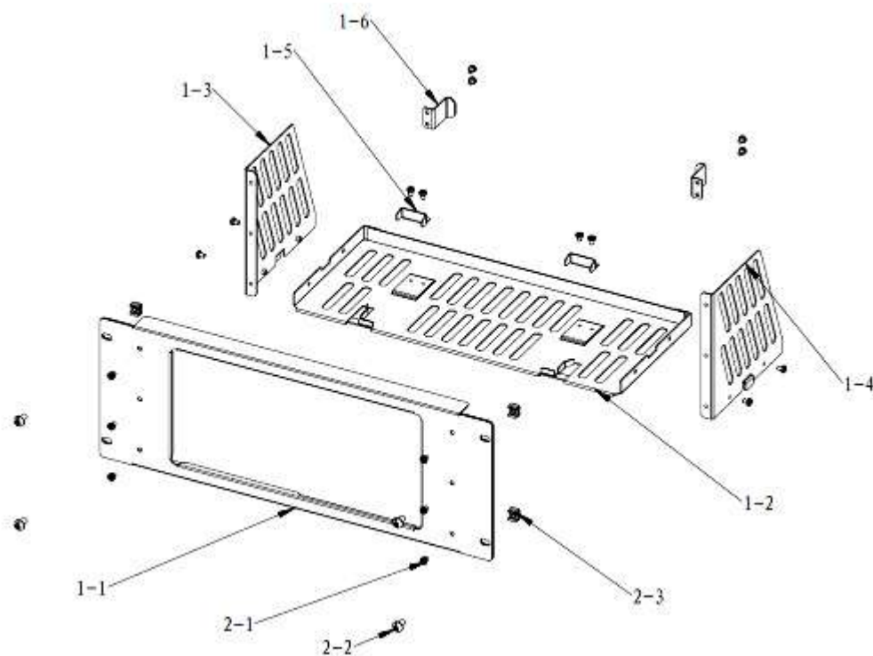
Bild 1-12 Teile Gestelleinbausatz
