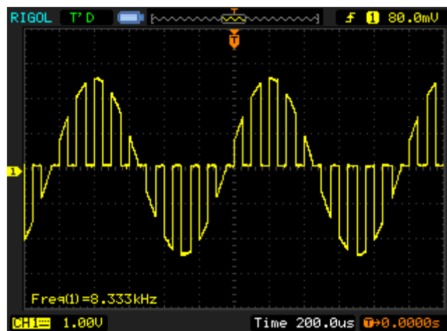
Bild 5-1 OSK-Moduliertes Signal
