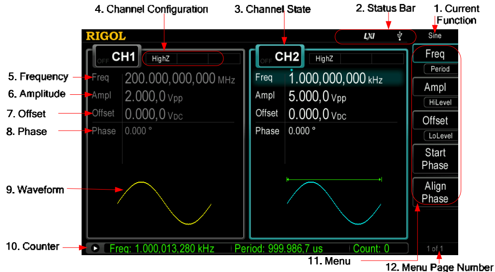
Bild 1-9 Benutzeroberfläche
